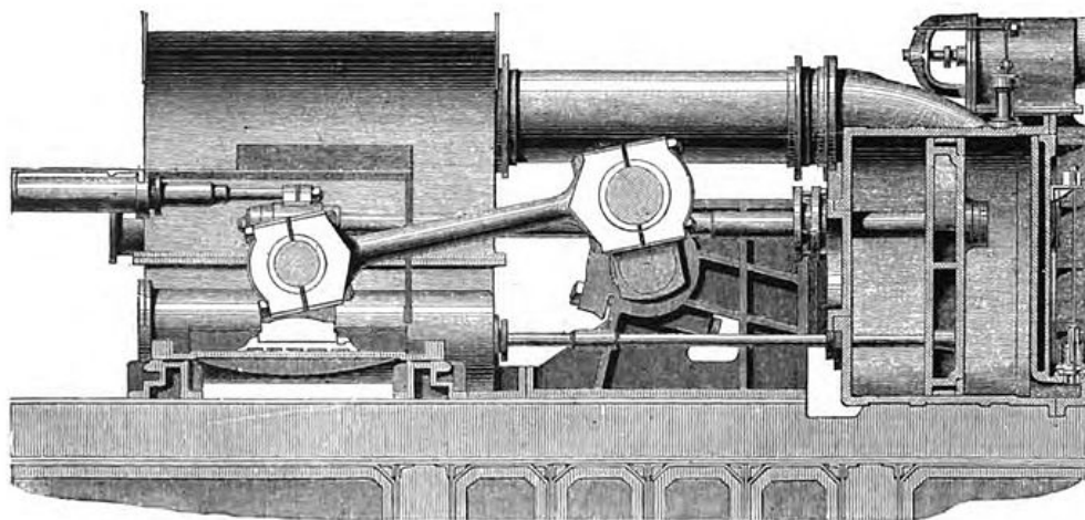
FIG. 12.—ENGINE OF H. M. S. AGINCOURT.
