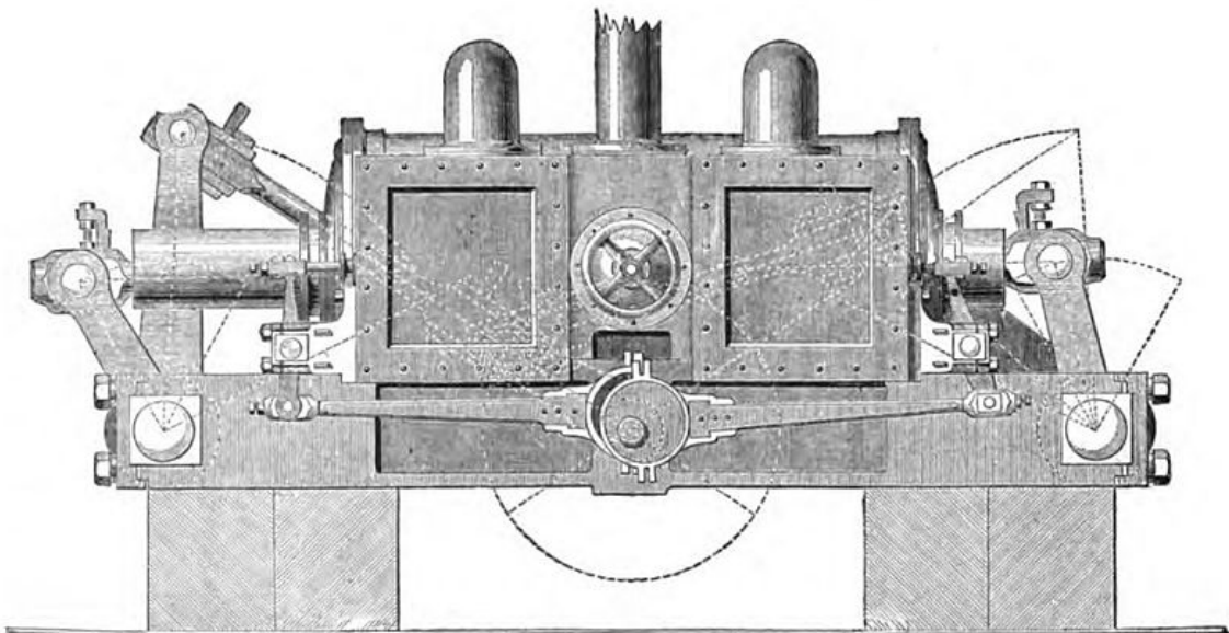
FIG. 38.—ENGINE OF U. S. MONITOR MONADNOCK.
