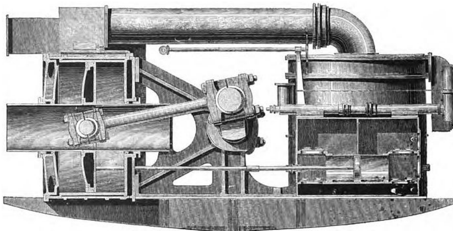
FIG. 10.—ENGINE OF H. M. S. BELLEROPHON.
